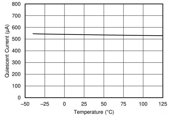
図 7-20. 静止電流と温度との関係
