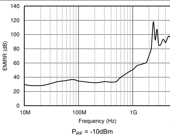
図 7-29. 非反転入力基準とする電磁干渉除去比 (EMIRR+) と周波数との関係 P_{RF} = -10\text{dBm}
