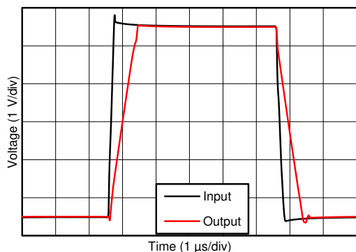
図 7-25. 過負荷からの回復
