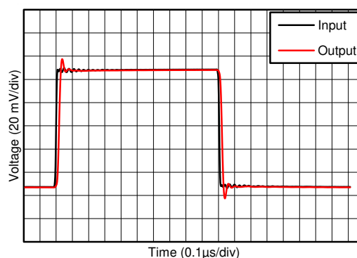
図 7-26. 小信号ステップ応答
