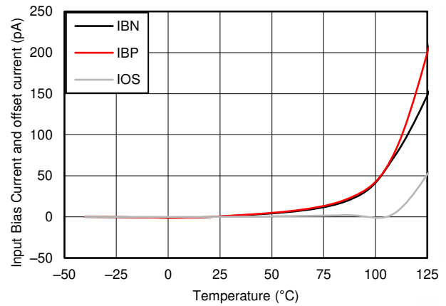
図 7-8. 入力バイアス電流と温度との関係
