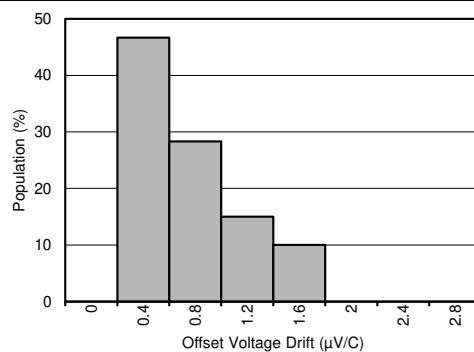
図 7-2. オフセット電圧ドリフトの分布
