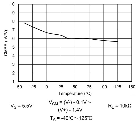
図 7-12. CMRR と温度との関係
