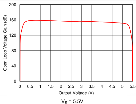
図 7-32. 開ループの電圧ゲインと出力電圧との関係
