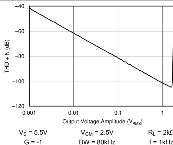
図 7-18. THD + N と振幅との関係
