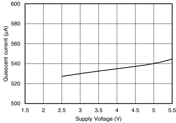
図 7-19. 静止電流と電源電圧との関係
