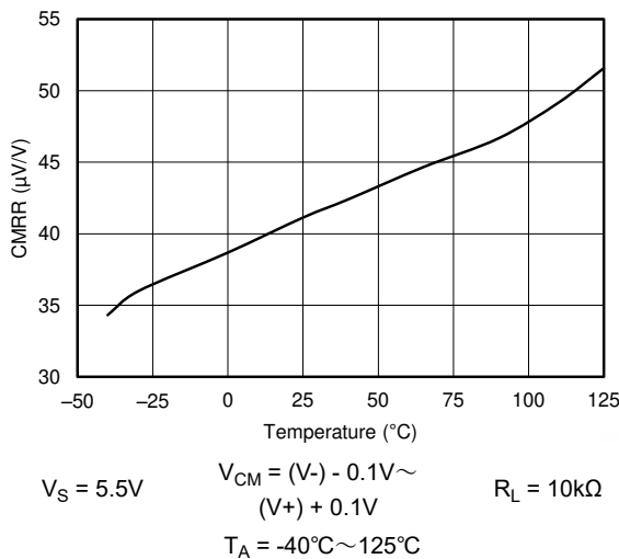
図 7-11. CMRR と温度との関係
