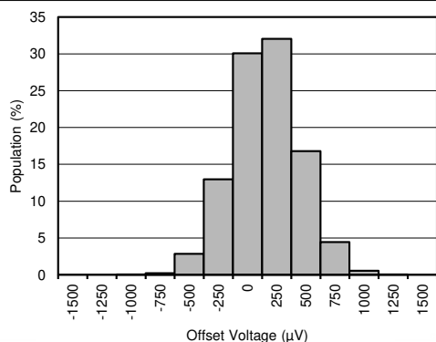
図 7-1. オフセット電圧の製造分布
