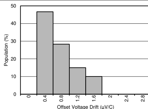
図 7-2. オフセット電圧ドリフトの分布
