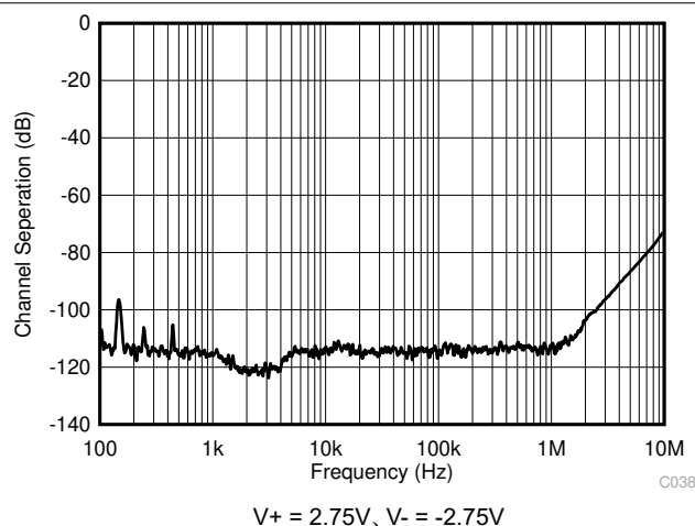
図 7-30. チャネル分離と周波数との関係 V_+ = 2.75\text{V} , V_- = -2.75\text{V}
