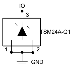
機能ブロック図
