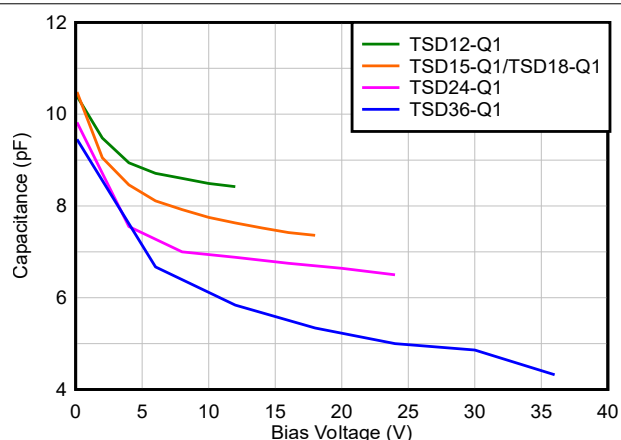
図 5-6. 静電容量とバイアス電圧との関係
