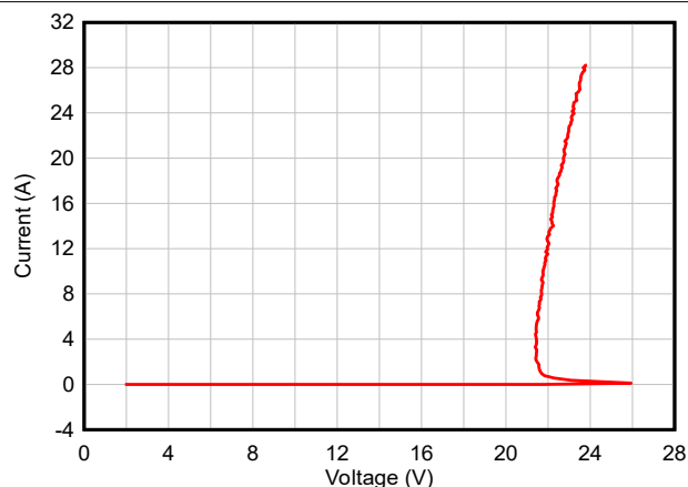
図 5-3. 正の TLP 曲線 - TSD18-Q1
