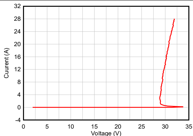
図 5-4. 正の TLP 曲線 - TSD24-Q1
