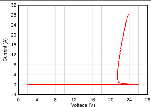
図 5-2. 正の TLP 曲線 - TSD15-Q1
