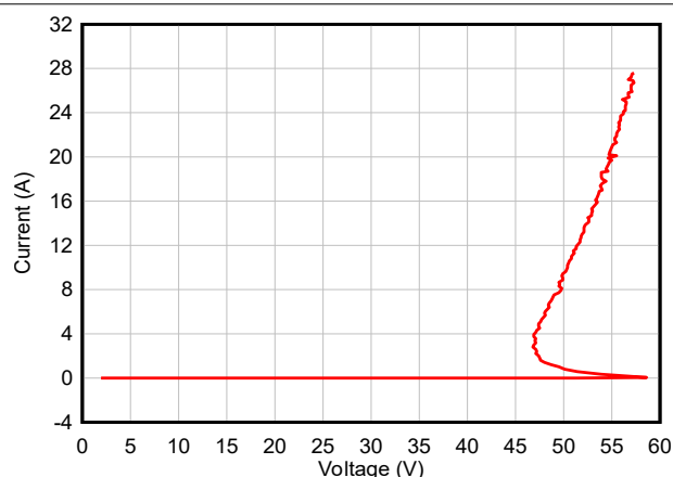
図 5-5. 正の TLP 曲線 - TSD36-Q1
