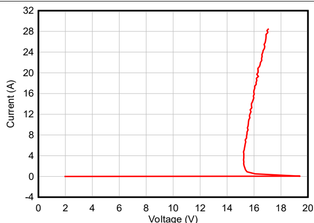
図 5-1. 正の TLP 曲線 - TSD12-Q1
