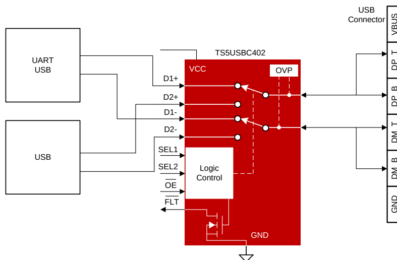
概略回路図
