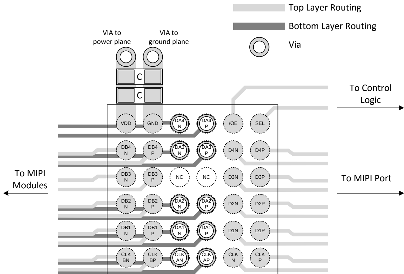
✕ 31. Layout Example
