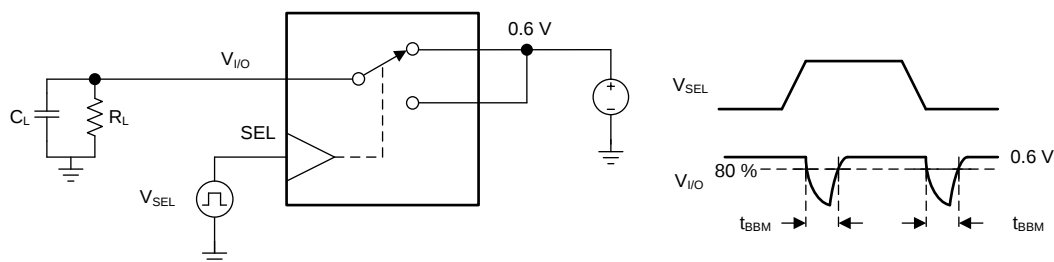
FIG 18. t_{SKEW}
