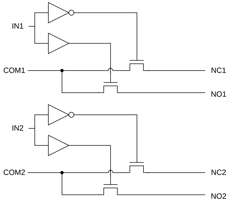
ブロック図
