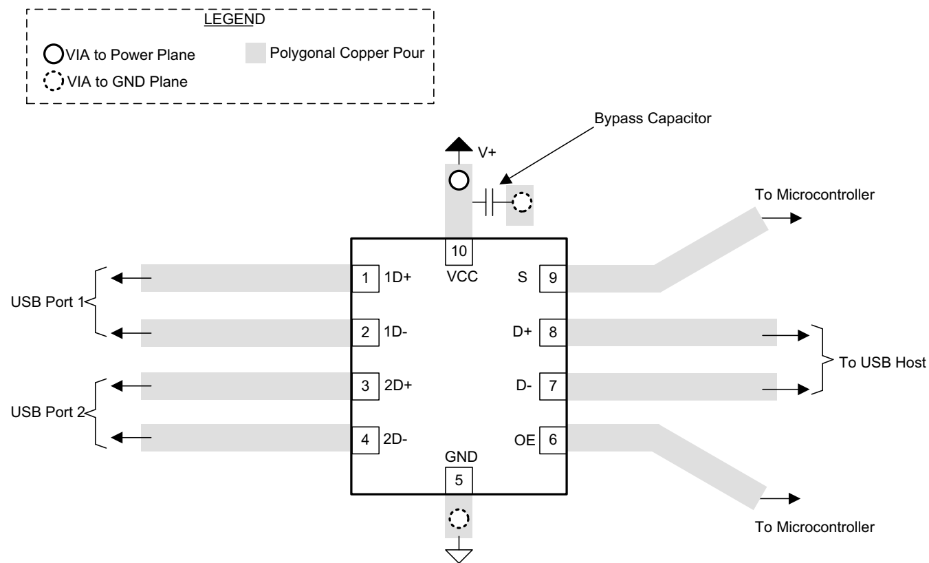
図 8-6. Package Layout Diagram
