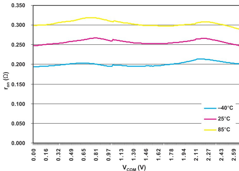
FIG 9-1. r_{ON} vs V_{COM}
