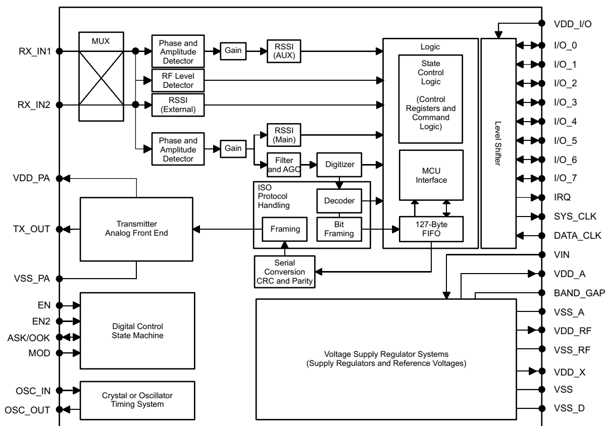
図 1-1. ブロック図
