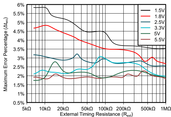
図 5-24. C_{ext} = 1\text{nF} での最大出力パルス幅誤差 (絶対値) とタイミング抵抗値との関係
