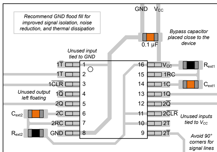
図 8-6. PW (TSSOP) パッケージの TPUL2T323-Q1 のプッシュプルレイアウト例
