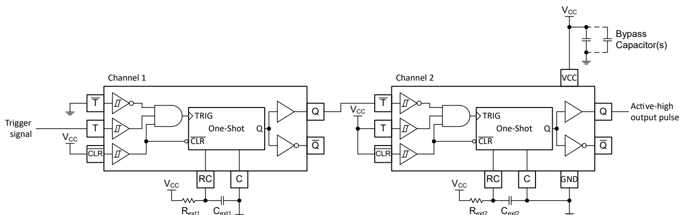
図 8-4. TPUL2T323-Q1 を使用した遅延パルス生成回路図
