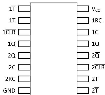
図 4-1. PW パッケージ 16 ピン TSSOP 上面図
