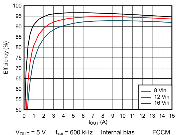
图 8-9. Efficiency
