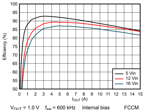
图 8-4. Efficiency
