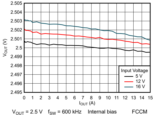
图 8-16. Load Regulation
