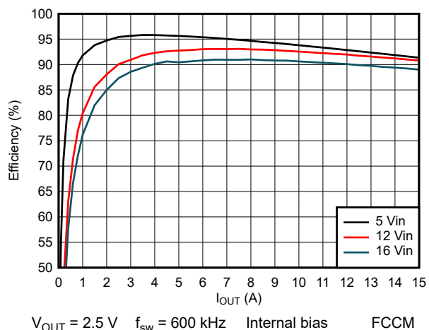
图 8-7. Efficiency
