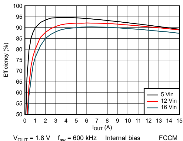
图 8-6. Efficiency
