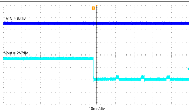
図 8-10. 通常動作から出力のハード短絡
