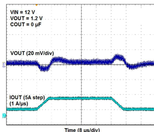
過渡応答
