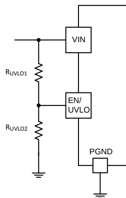
図 16. Adjustable UVLO
