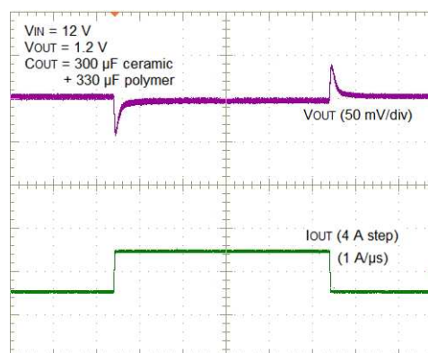
過渡応答
