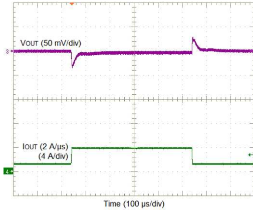
図 15. V_{OUT} = 0.8\text{ V} , 3-A Load Step
