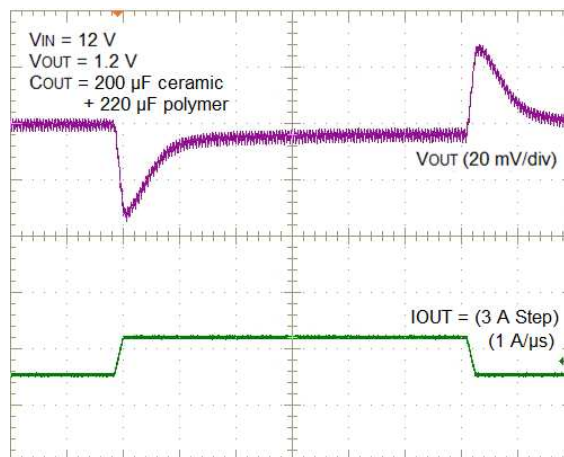
過渡応答
