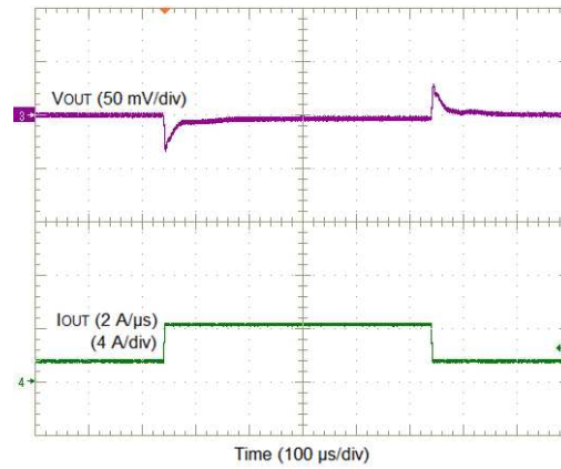
図 16. V_{OUT} = 0.8\text{ V} , 3-A Load Step
