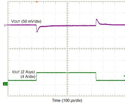
図 16. V_{OUT} = 0.8\text{ V} , 3-A Load Step
