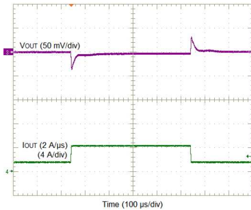
図 15. V_{OUT} = 0.8\text{ V} , 3-A Load Step
