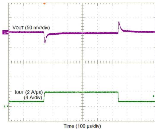
図 17. V_{OUT} = 1\text{ V} , 3-A Load Step
