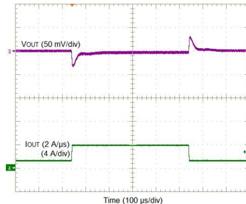
図 18. V_{OUT} = 1\text{ V} , 3-A Load Step
