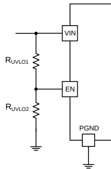
图 20. Adjustable UVLO
