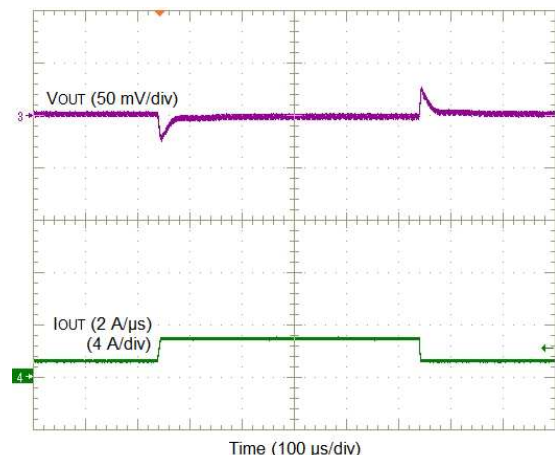
図 17. V_{OUT} = 1\text{ V} , 2-A Load Step
