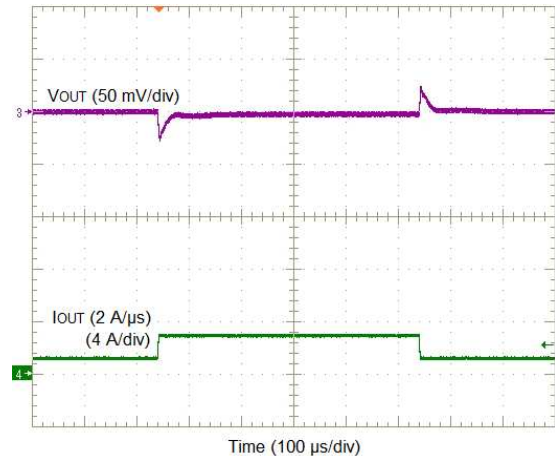
図 15. V_{OUT} = 0.8\text{ V} , 2-A Load Step
