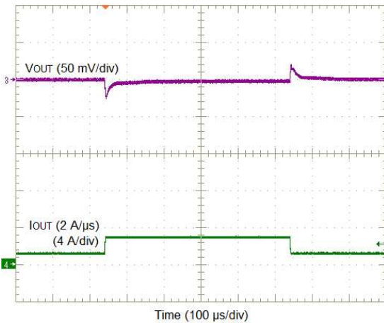
図 14. V_{OUT} = 0.8\text{ V} , 2-A Load Step
