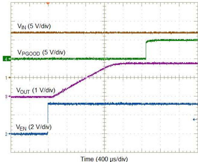
13. Enable Turnon
