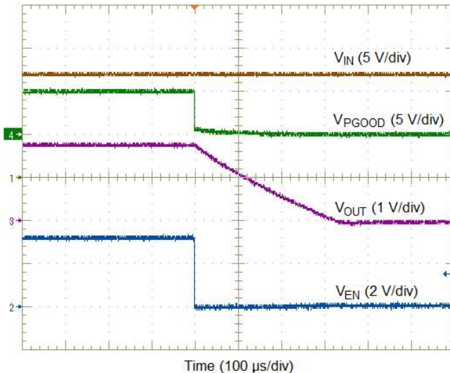
12. Enable Turnoff
