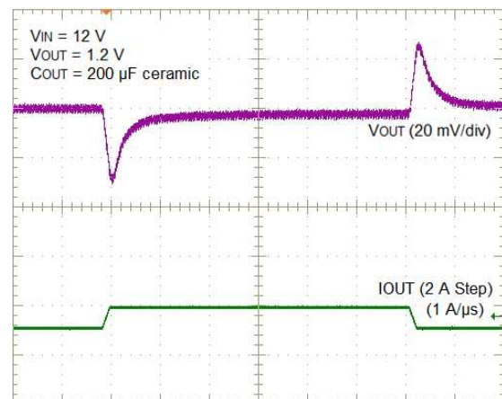
過渡応答
