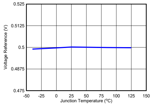
図 6-6. V_{REF}
