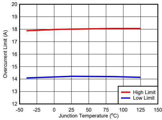
図 6-3. Overcurrent Limit
