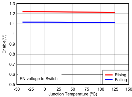
図 6-5. Enable Voltage
