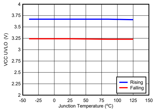
図 6-8. V_{CC} UVLO
