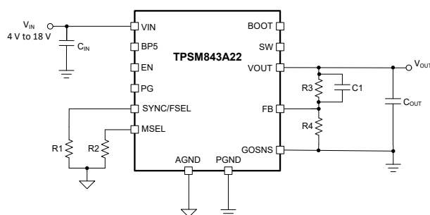
TPSM843A22 のアプリケーション概略図
