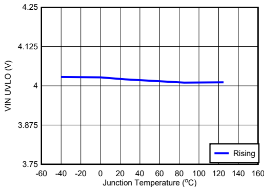
図 6-7. V_{IN} UVLO
