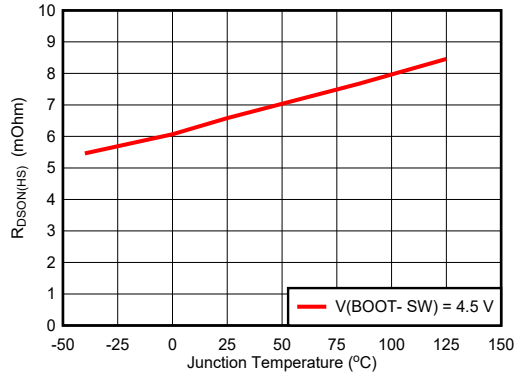
図 6-1. High-Side FET R_{DS(ON)}
