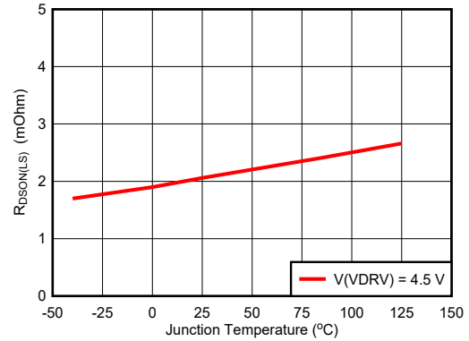
図 6-2. Low-Side FET R_{DS(ON)}
