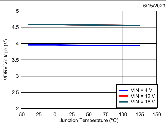
图 6-15. VDRV vs Temperature
