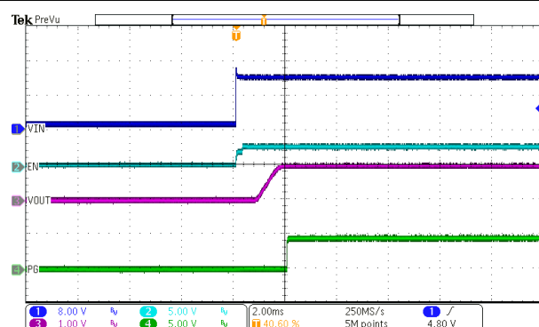
図 7-11. EN Start-Up – With Load
