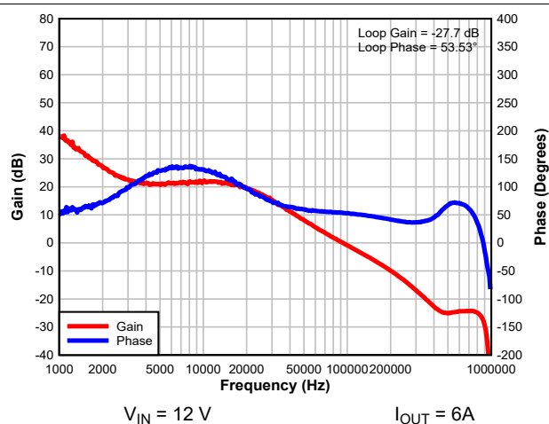
図 7-7. Bode Plot
