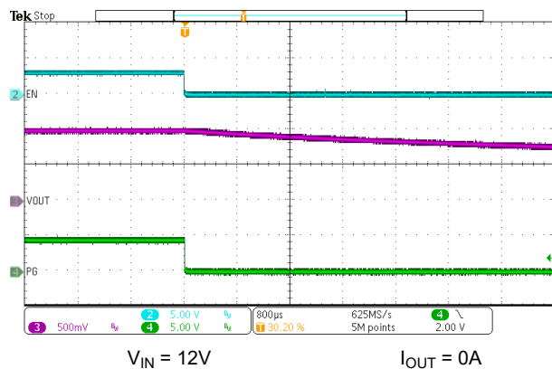
7-10. EN Shutdown No Load
