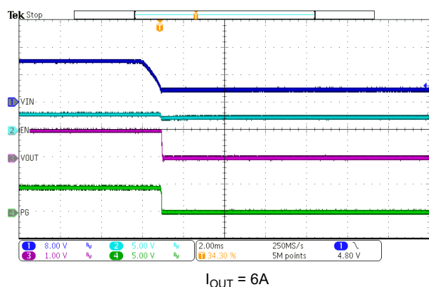
7-14. VIN Shutdown
