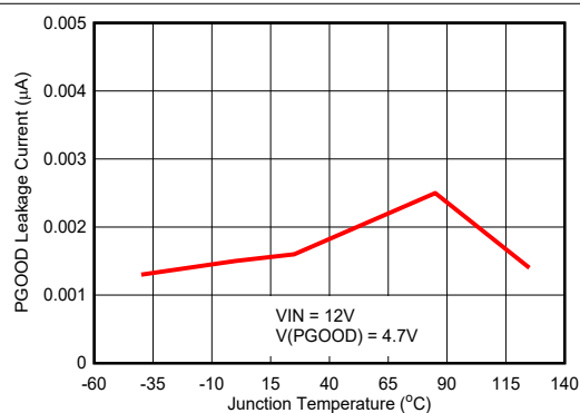
図 5-10. PG Leakage
