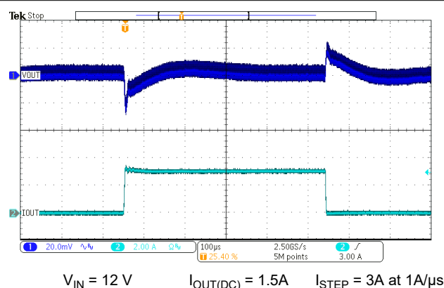
図 7-8. Load Transient
