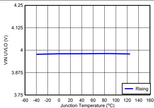
図 5-8. Vin UVLO
