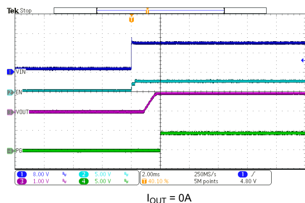
図 7-13. VIN Start-Up
