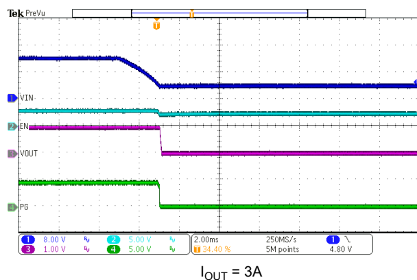
図 7-14. VIN Shutdown
