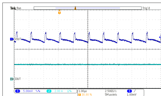
図 7-16. Output Ripple – 3A Load
