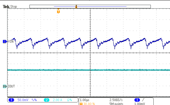
図 7-17. Input Ripple – No Load
