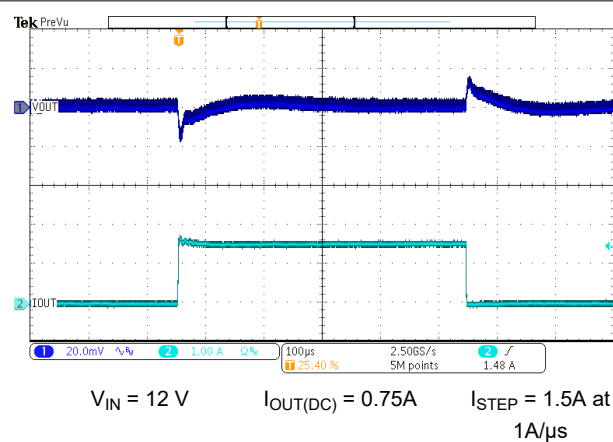
図 7-8. Load Transient
