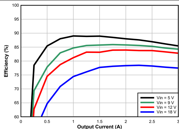
図 7-4. Efficiency
