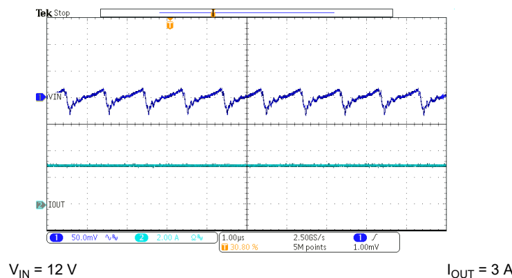
図 7-18. Input Ripple – 3-A Load
