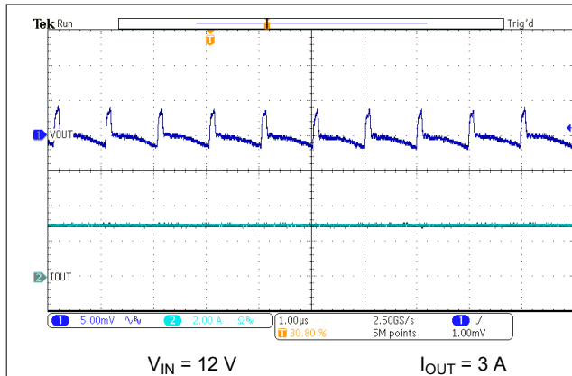
図 7-16. Output Ripple – 3-A Load
