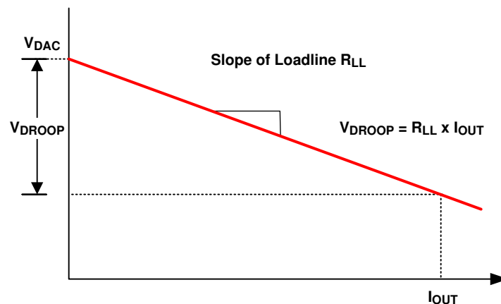
图 7-3. Load Line
