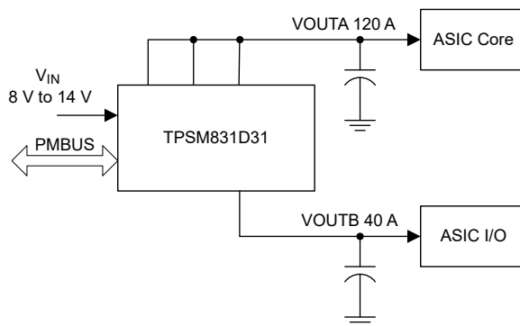
簡素化されたアプリケーション
