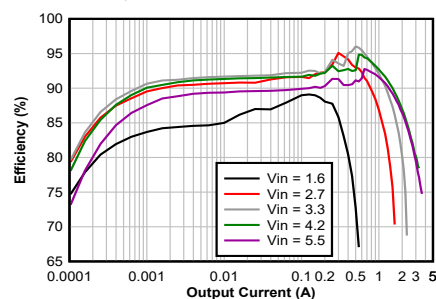
効率と出力電流との関係 ( V_{OUT} = 3.3V )
