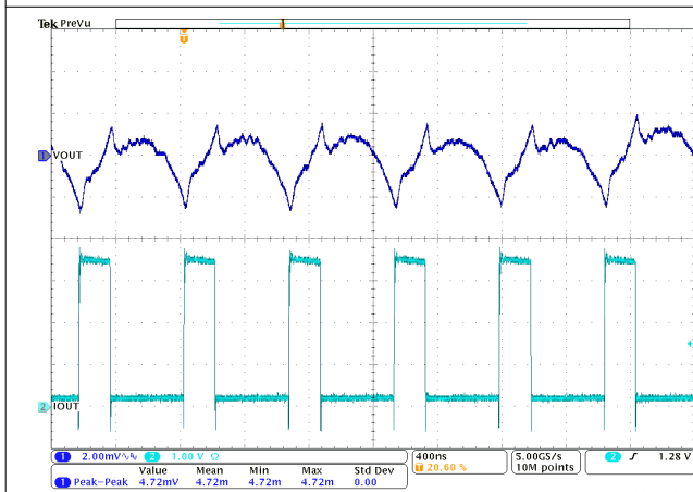
図 9-20. 負荷過渡 TPSM8287B30xx
