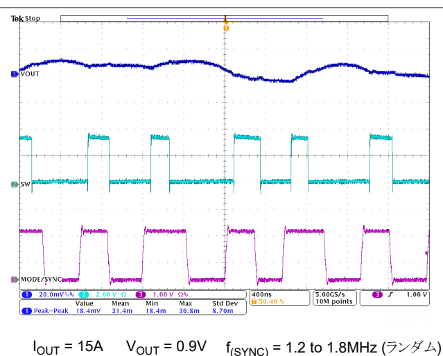
図 9-27. ランダムな外部クロックへの同期
