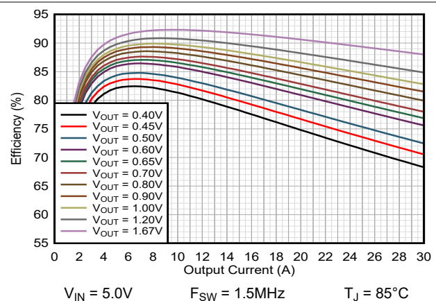
図 9-7. 効率 TPSM8287B30xx FPWM
