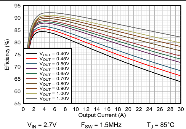
図 9-3. 効率 TPSM8287B30xx FPWM
