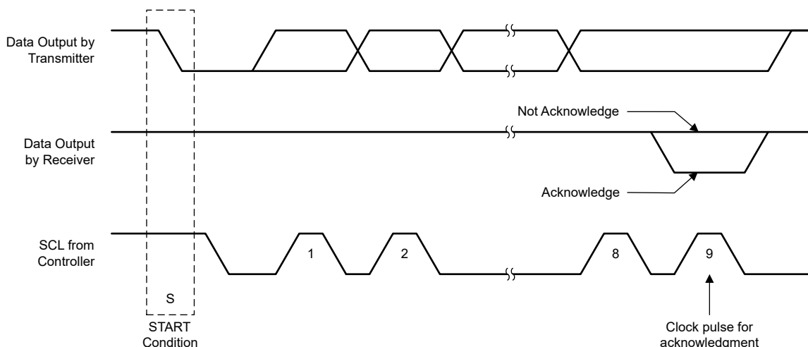
図 7-20. I²C バスのアクノリッジ
