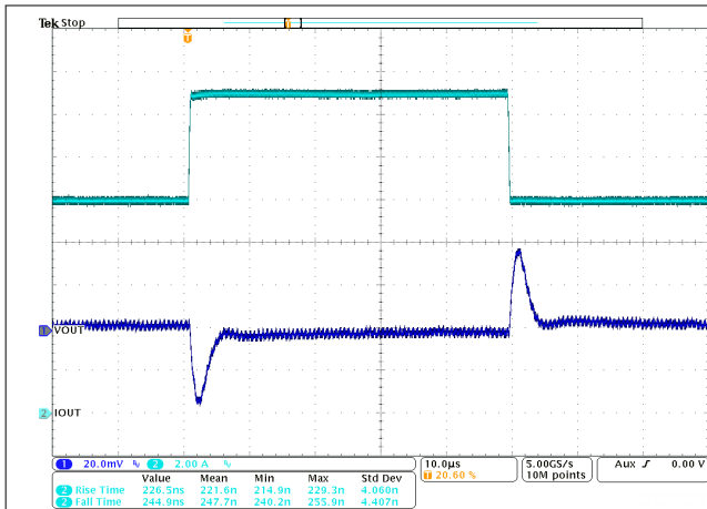
図 9-20. 負荷過渡 TPSM8287B30xx
