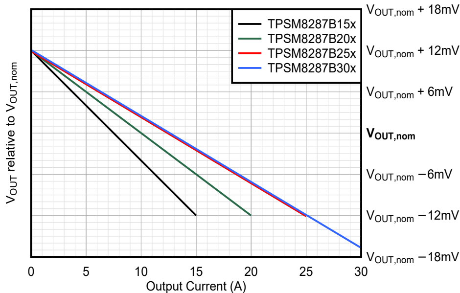
図 7-10. 出力電流による電圧スケーリング
