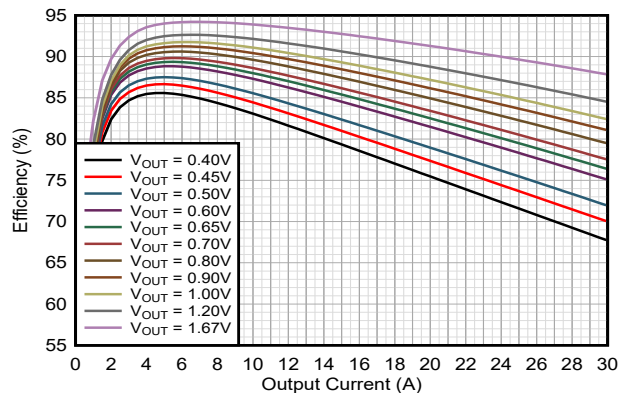
効率性 TPSM8287B30x ( V_{IN} = 3.3V 、FPWM)
