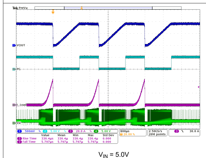
図 9-28. 電流制限 (ヒカップ = 1)
