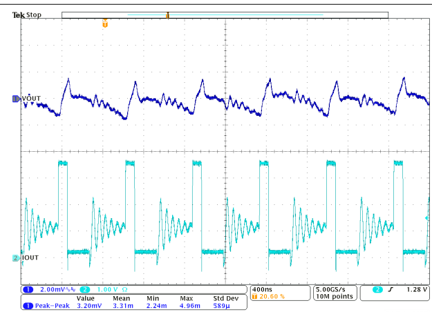
図 9-21. 負荷過渡 TPSM8287B30xx
