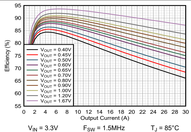
図 9-5. 効率 TPSM8287B30xx FPWM
