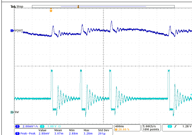
図 9-22. PWM-CCM 動作 TPSM8287B30xx
