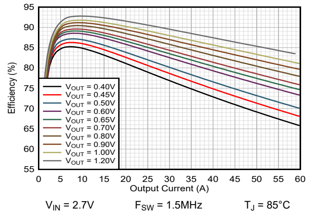
図 9-38. 効率 TPSM8287B30xx FPWM
