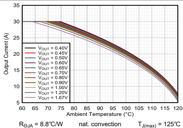
図 9-32. 安全動作領域 TPSM8287B30xx V_{IN} = 3.3V
