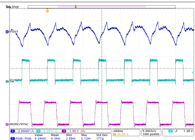
図 9-23. PWM-DCM 動作 TPSM8287B30xx
