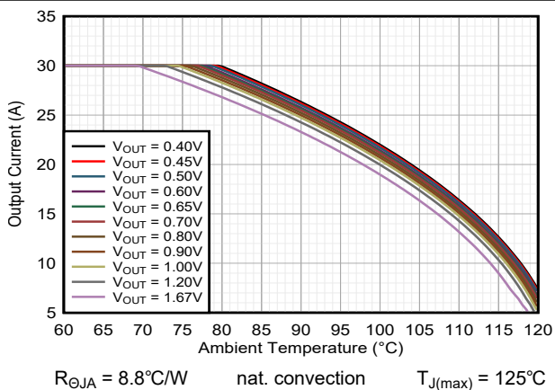
図 9-33. 安全動作領域 TPSM8287B30xx V_{IN} = 5.0V
