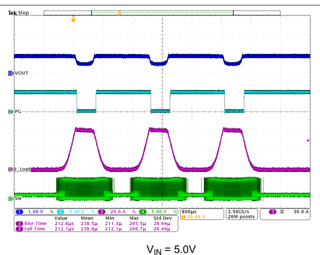
図 9-29. 電流制限 (ヒカップ = 0)
