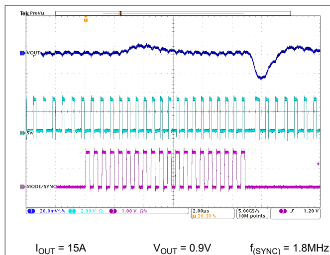
図 9-26. 外部クロックの追加と取り外し
