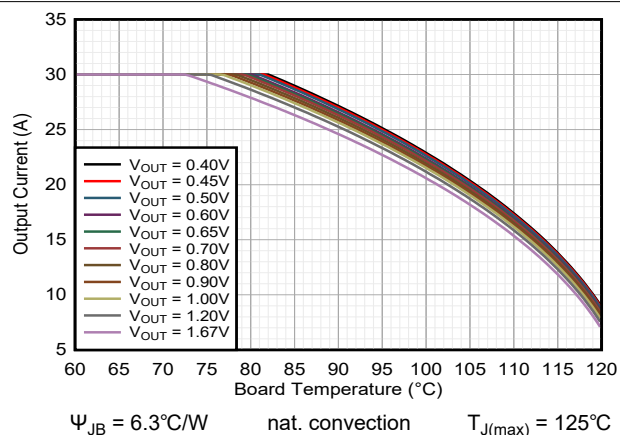
図 9-34. 安全動作領域 TPSM8287B30xx V_{IN} = 3.3V
