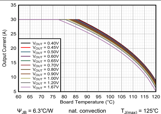
図 9-35. 安全動作領域 TPSM8287B30xx V_{IN} = 5.0V
