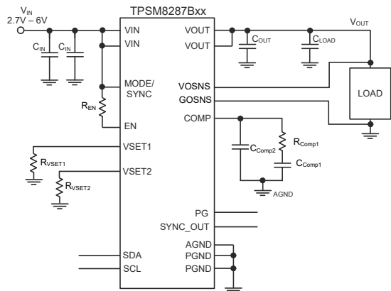
TPSM8287Bxx の概略回路図
