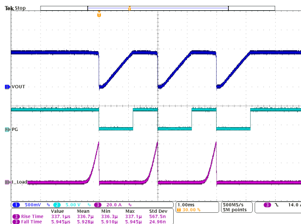
図 7-14. ヒカップ電流制限
