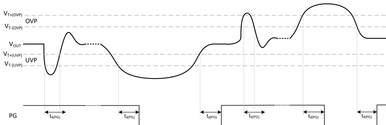
図 7-15. パワー グッドの過渡応答と遅延動作
