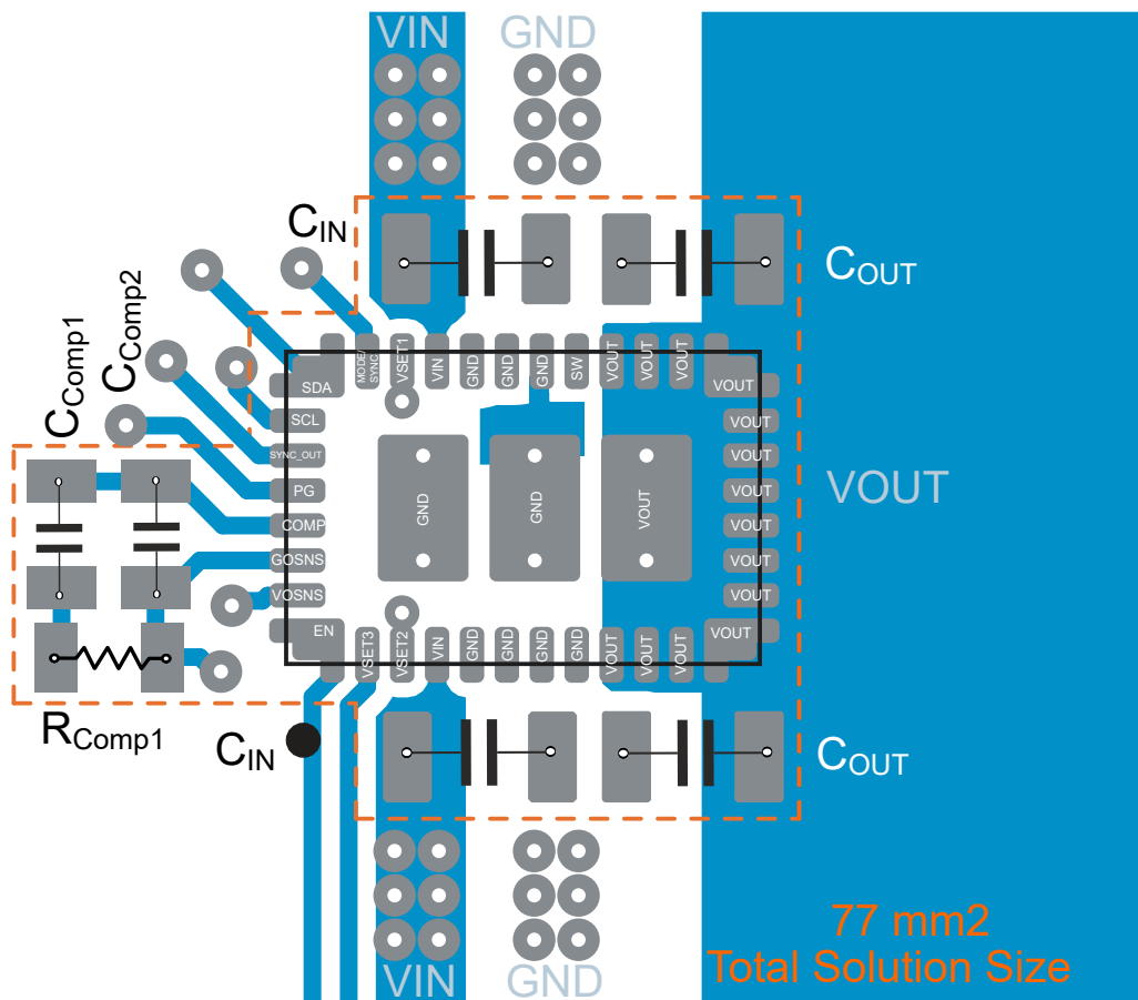
図 9-47. Layout Example
