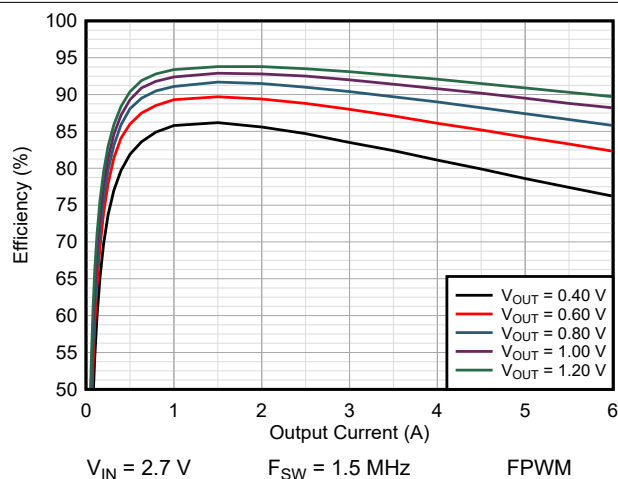
図 9-2. Efficiency TPSM8287A06BAS
