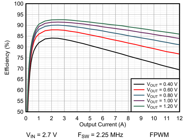
図 9-9. Efficiency TPSM8287A12BBS
