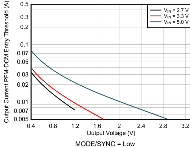
図 7-5. PFM-DCM Entry Threshold TPSM8287A06BAS
