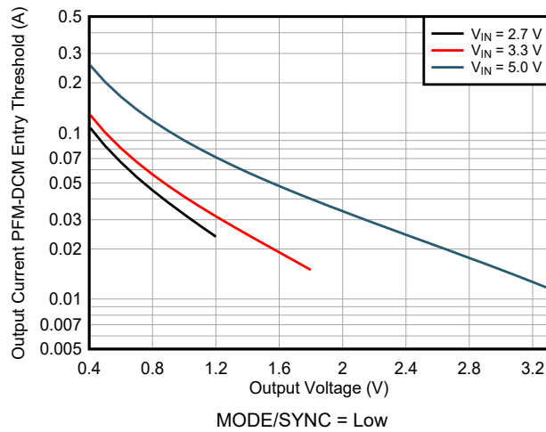
図 7-7. PFM-DCM Entry Threshold TPSM8287A12BBS
