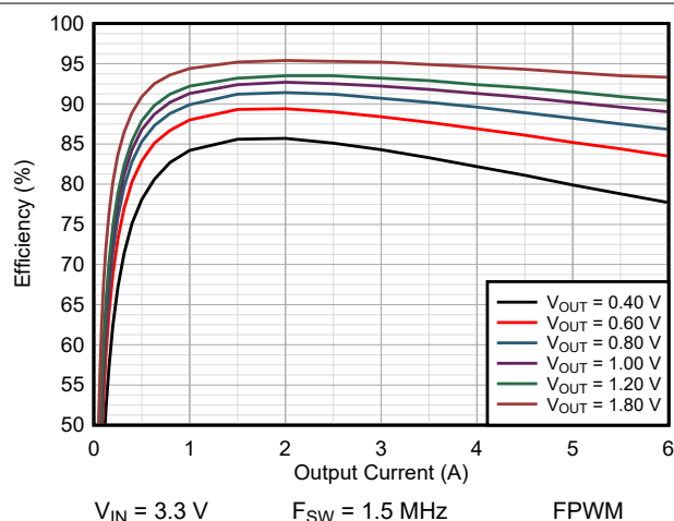
図 9-4. Efficiency TPSM8287A06BAS
