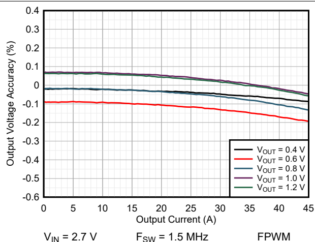
図 9-52. Load Regulation
