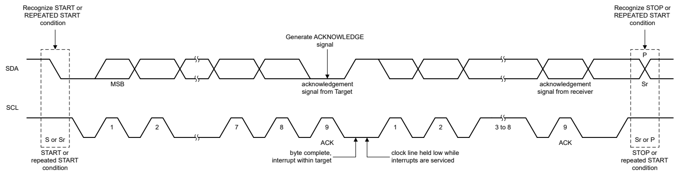
図 7-26. Bus Protocol
