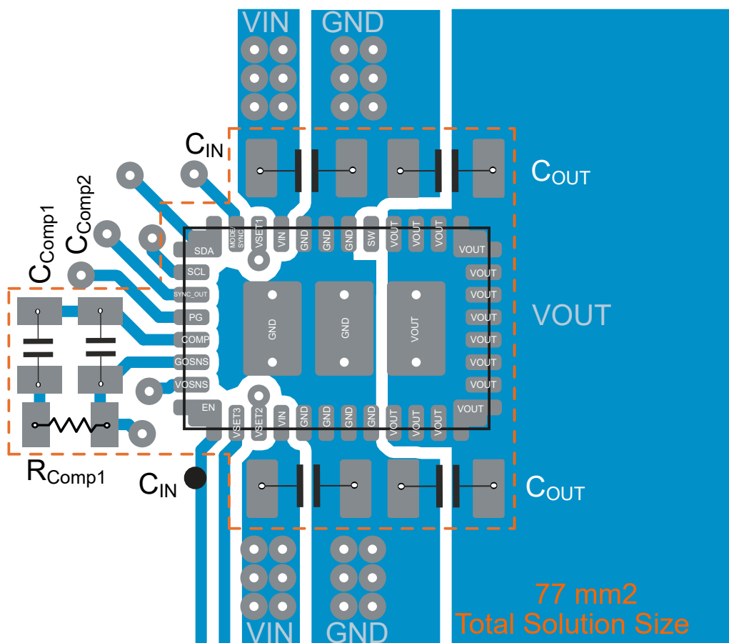
図 9-57. Layout Example
