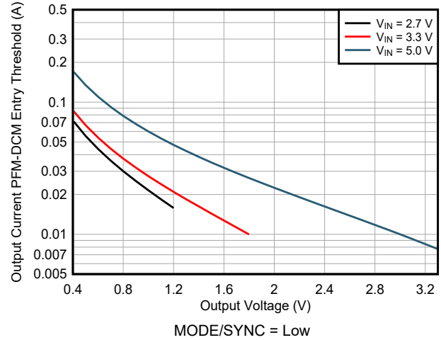
図 7-6. PFM-DCM Entry Threshold TPSM8287A12BAS
