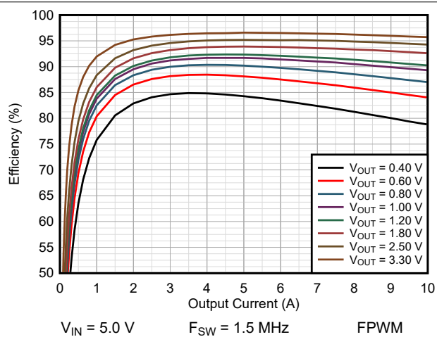
図 9-7. Efficiency TPSM8287A10BAH
