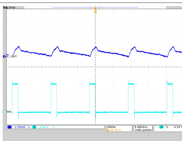
図 9-27. PWM-CCM Operation TPSM8287A12BBS
