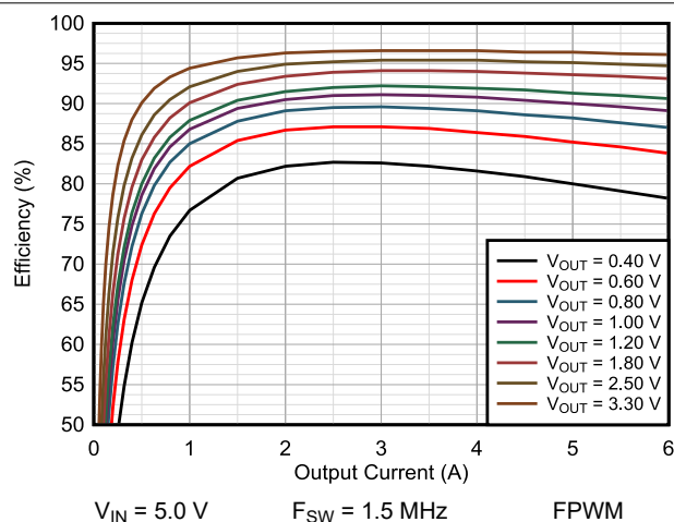
図 9-6. Efficiency TPSM8287A06BAS
