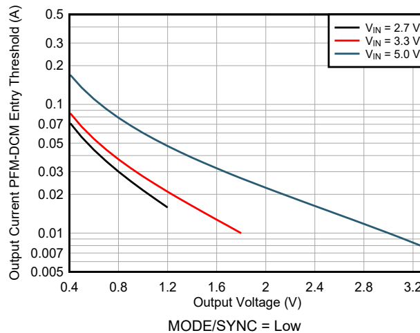
図 7-9. PFM-DCM Entry Threshold TPSM8287A15BBH
