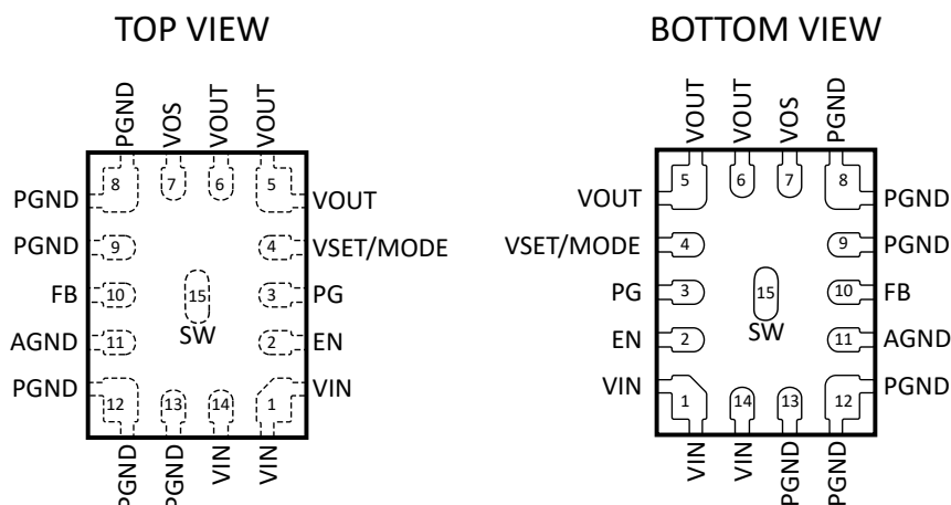
図 5-1. TPSM82864A, TPSM82866A - RCF (15 Pin) QFN-FCMOD
