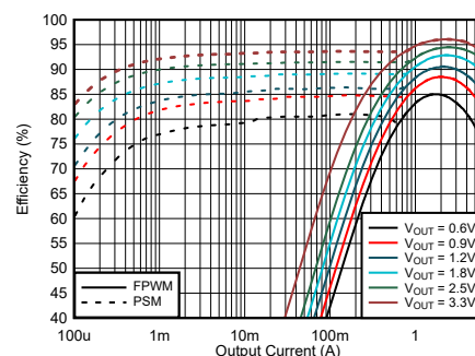
TPSM82864AA0HRDMR – 効率と出力電流との関係、 V IN = 5.0V
