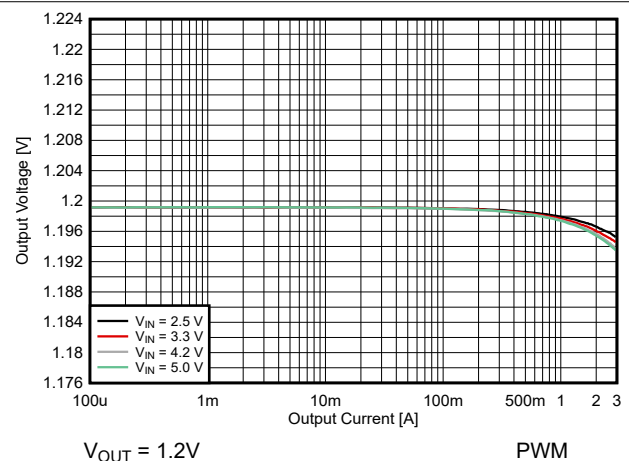
図 8-19. 出力電圧と出力電流との関係
