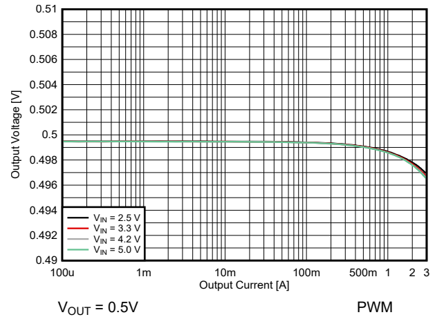
図 8-15. 出力電圧と出力電流との関係
