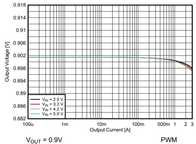
図 8-17. 出力電圧と出力電流との関係
