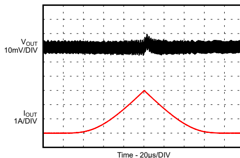
9-156. Load Sweep
