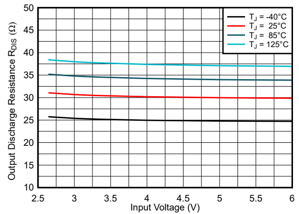
図 6-4. Discharge Resistance
