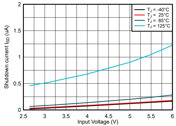
図 6-2. Shutdown Current
