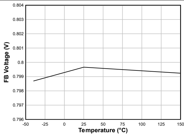
図 6-1. Feedback Voltage
