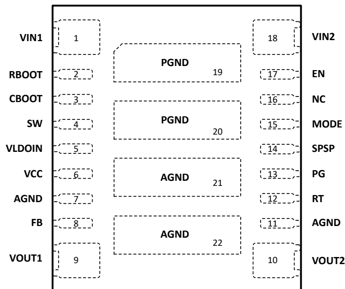
図 5-1. 22-Pin B3QFN RDF Package (Top View)
