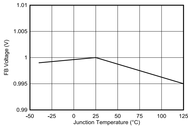
図 6-3. Feedback Voltage
