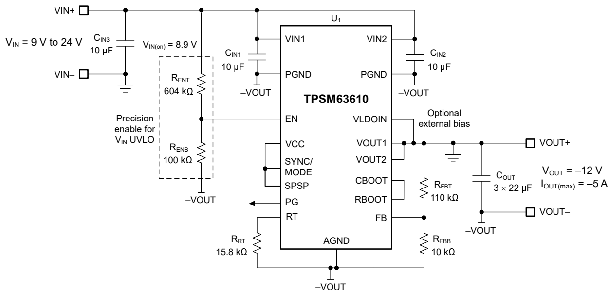
図 8-14. Circuit Schematic
