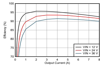
代表的な効率、 V_{OUT} = 5V 、 F_{SW} = 1MHz
