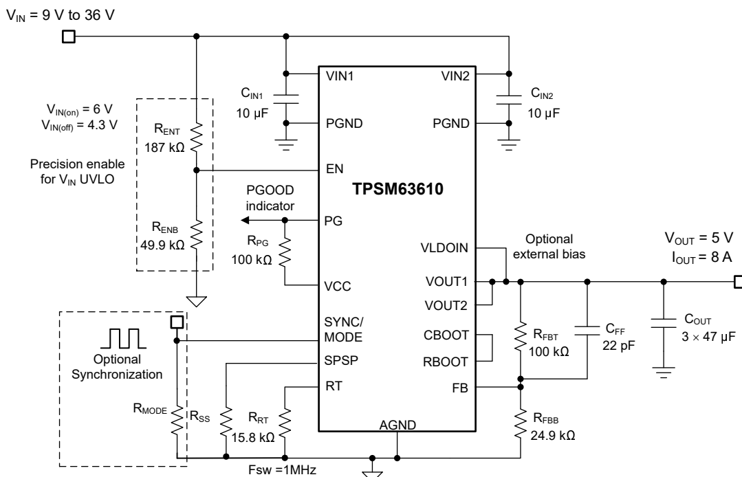
図 8-1. Circuit Schematic
