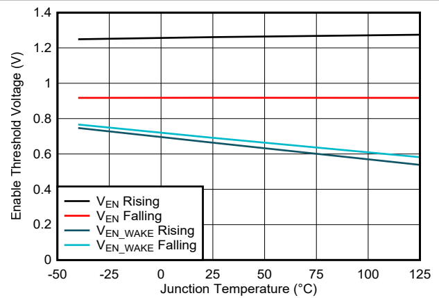
図 6-6. Enable Thresholds
