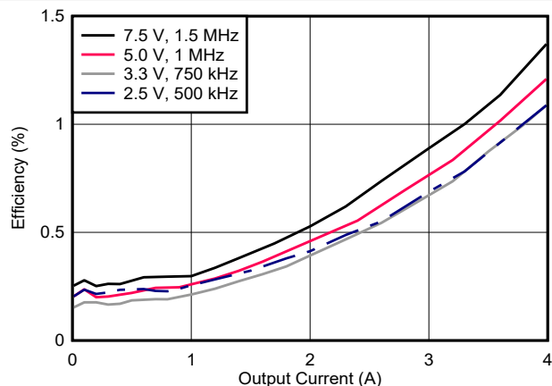
図 7-10. Power Dissipation
