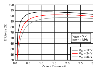
代表的な効率 (V OUT = 5V、f SW = 1MHz)
