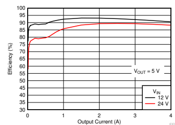
5V OUT の効率
