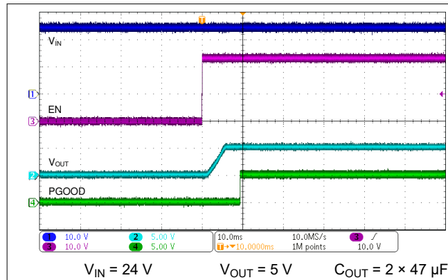
8-2. Enable Turn-ON
