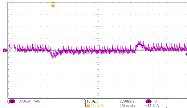
8-4. 5-A Transient Load Step
