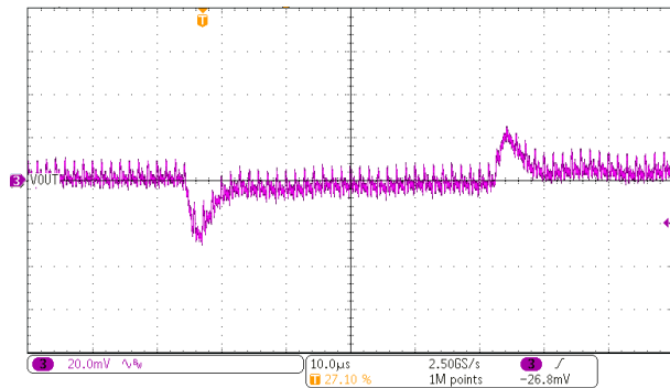
8-5. 10-A Transient Load Step
