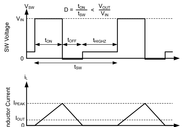
図 9-13. PFM Operation
