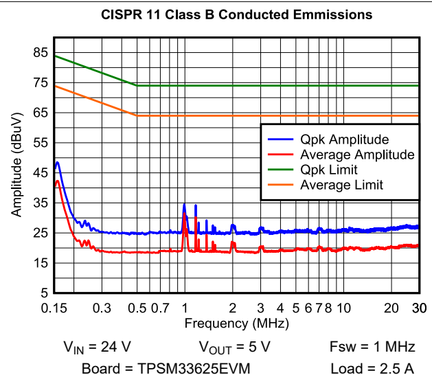
図 8-20. CISPR 11, Class B, CE Scan 150 kHz–30 MHz
