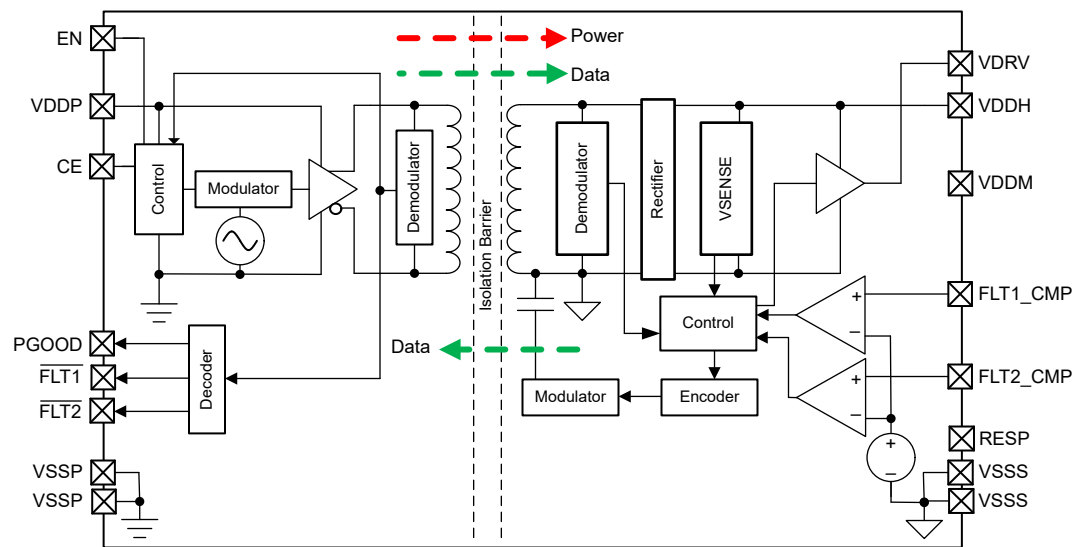
图 8-2. TPSI311x, TPSI311xL
