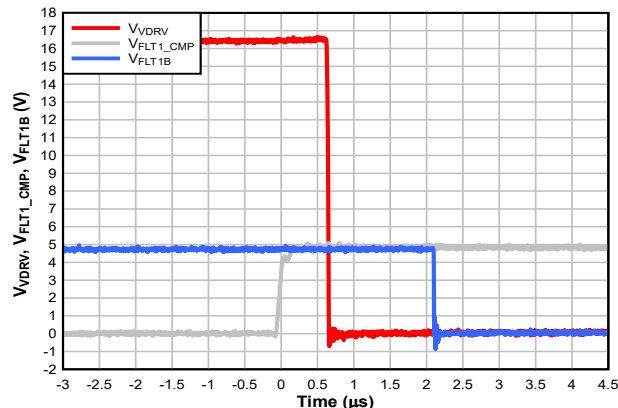
図 6-9. t_{\text{HL\_VDRV\_CE}} (zoomed out)
