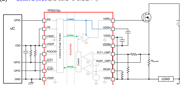
TPSI3100 の概略回路図
