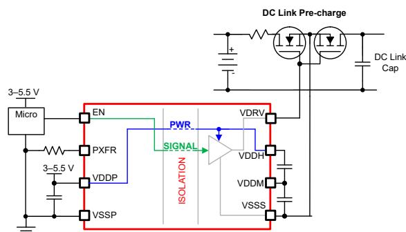
TPSI3052 の概略回路図
