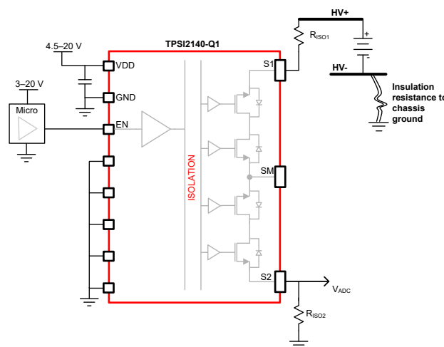
TPSI2140-Q1 アプリケーション概略回路図
