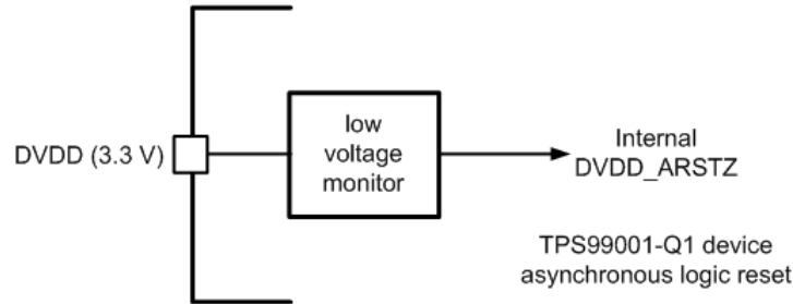
図 6-2. Internal DVDD Monitor
