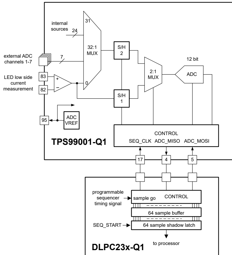
図 6-1. ADC Subsystem Block Diagram
