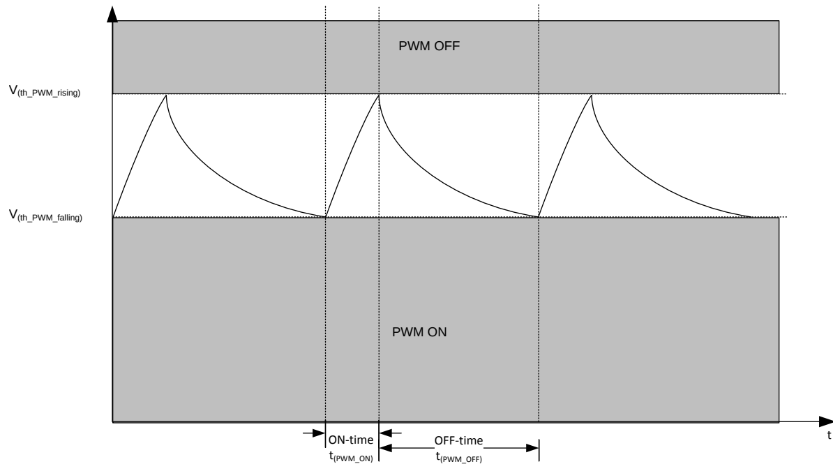
图 24. PWM Dimming Profile
