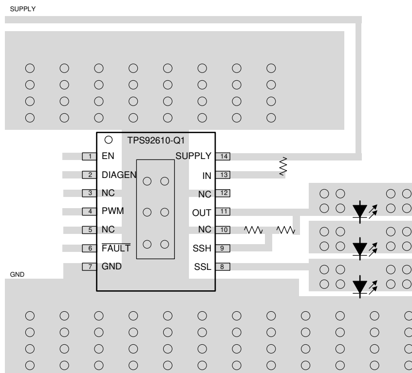
FIG 27. TPS92610-Q1 Example Layout Diagram
