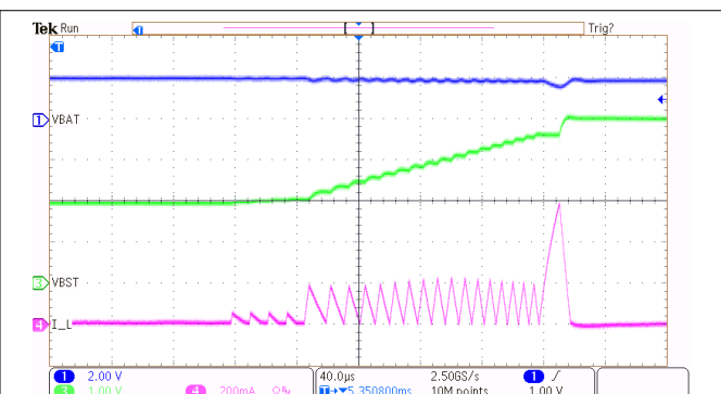
图 9-3. Boost Soft-Start
